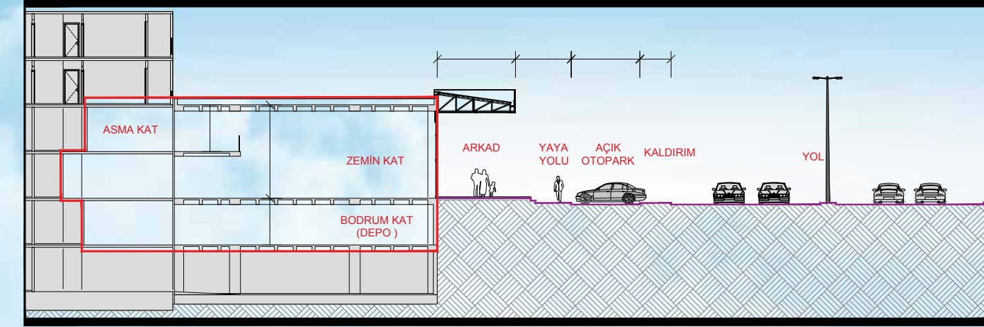
ÖRNEK DÜKKAN KESİTİ
